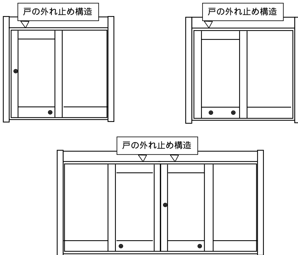
図6 ガラス引戸（自動を含む）の構造例
