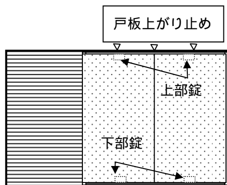
図 1 1 雨戸の構造例
