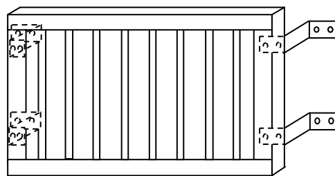
図12-3 面格子を躯体にブラケットにより取付ける場合の構造例
