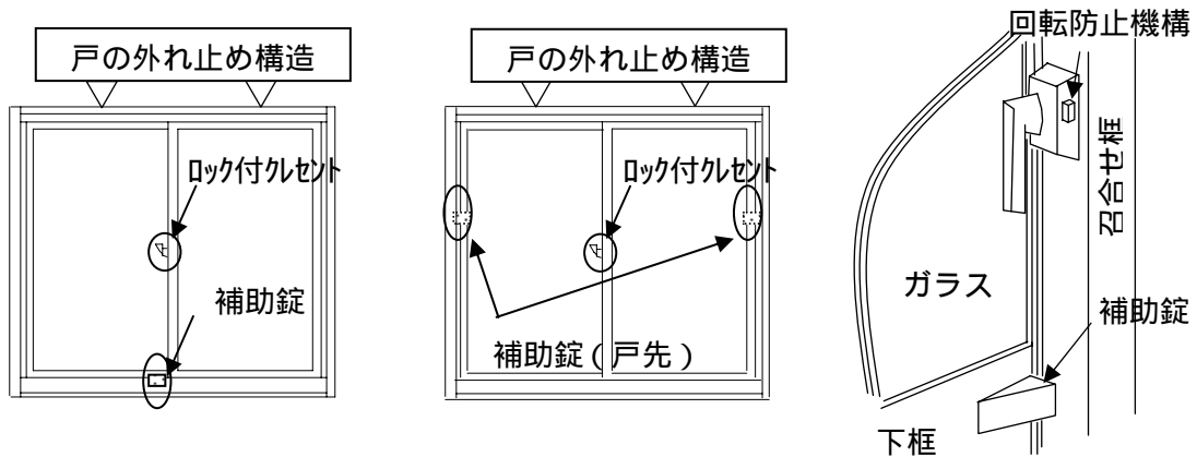
図7 引き形式のサッシの構造例
