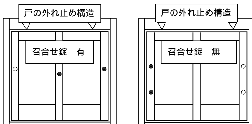
図5 引戸の構造例
