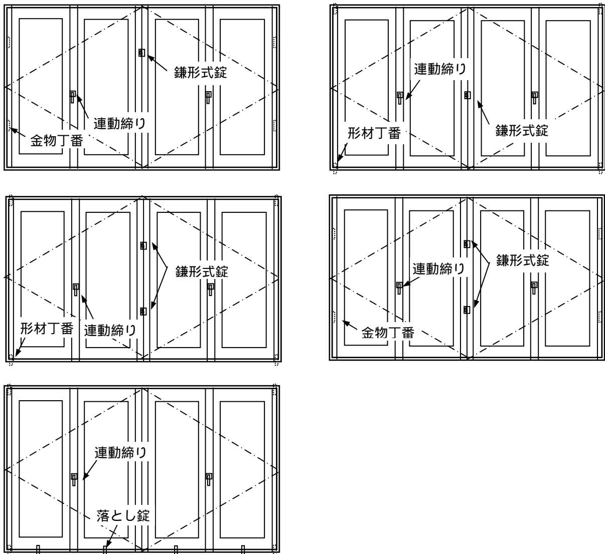
図9 折りたたみ形式のサッシの構造例
