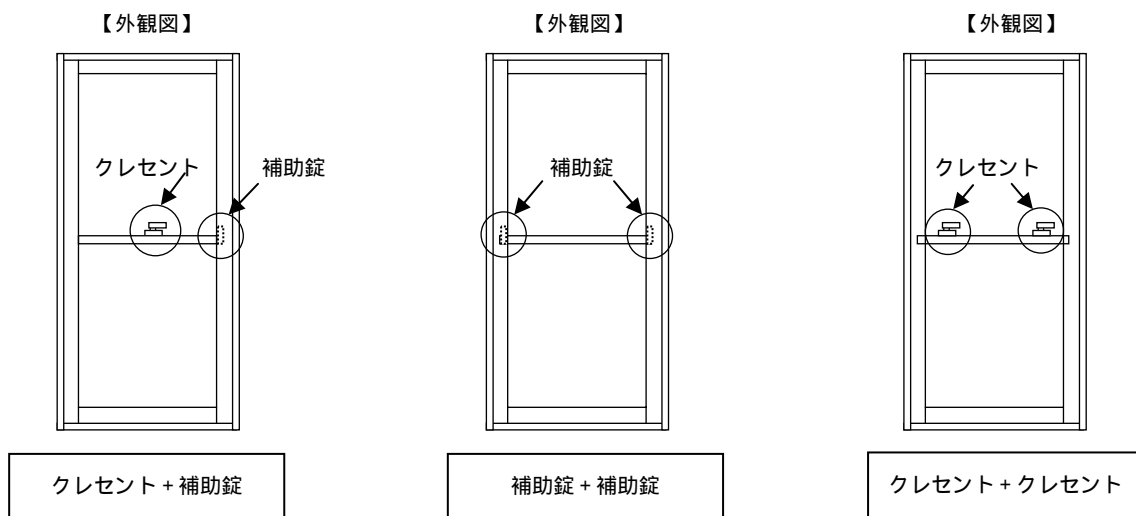
図4 - 2 上げ下げ内蔵ドア 可動障子部の構造例
