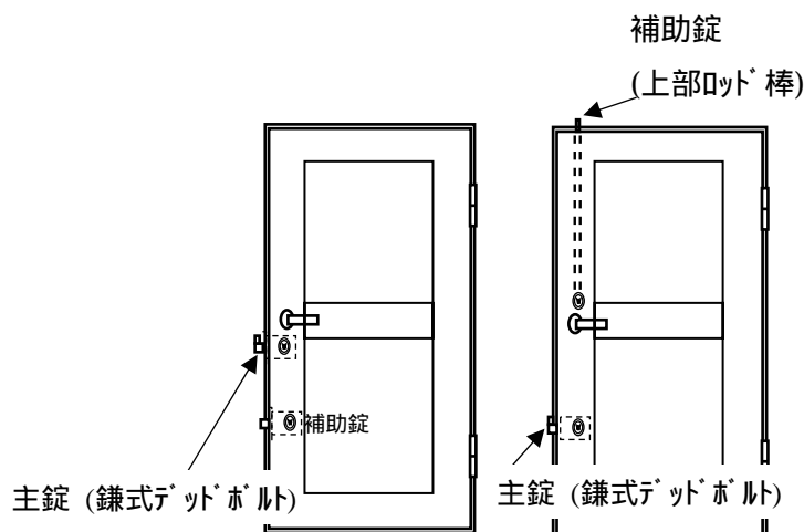
図3 ガラスドアの構造例
