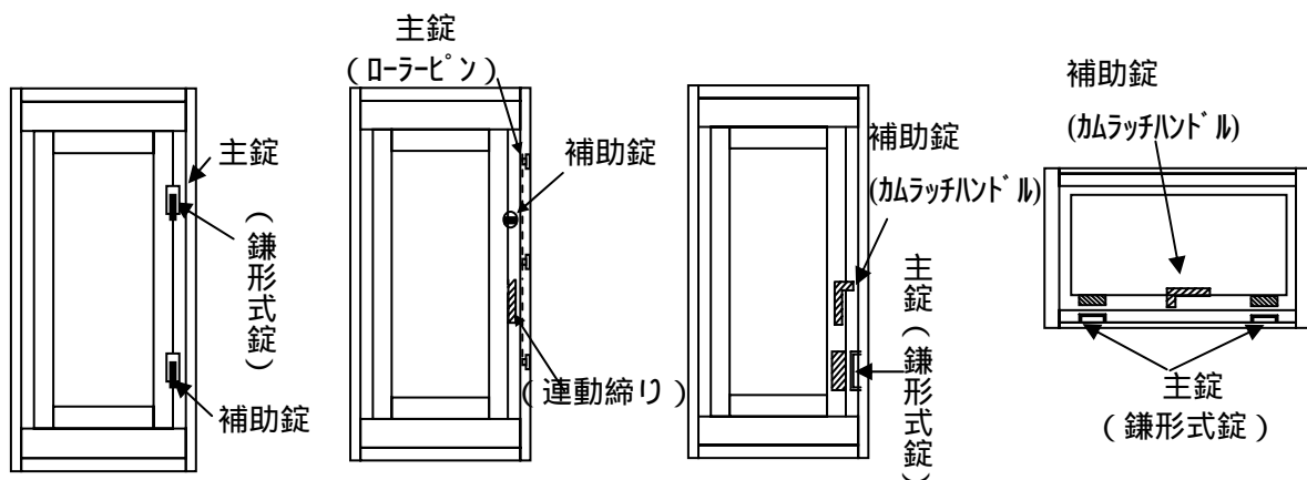
図8 開き形式のサッシの構造例
