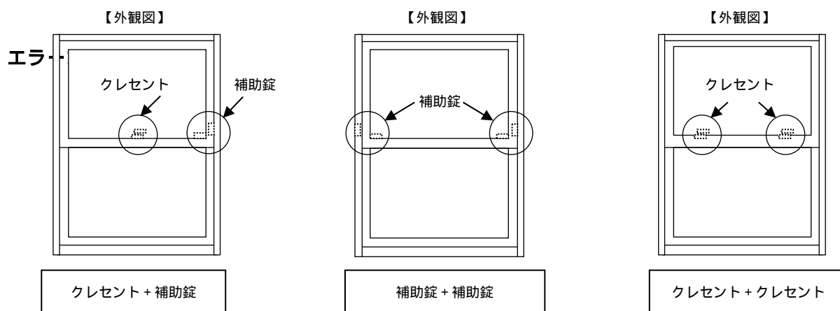
図10 上げ下げ形式のサッシの構造例
