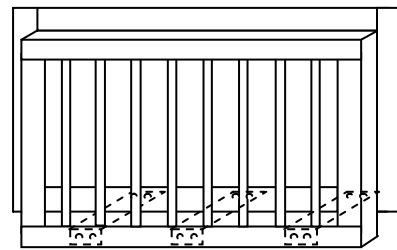
図12-2 面格子をサッシ枠に取付ける場合の構造例
