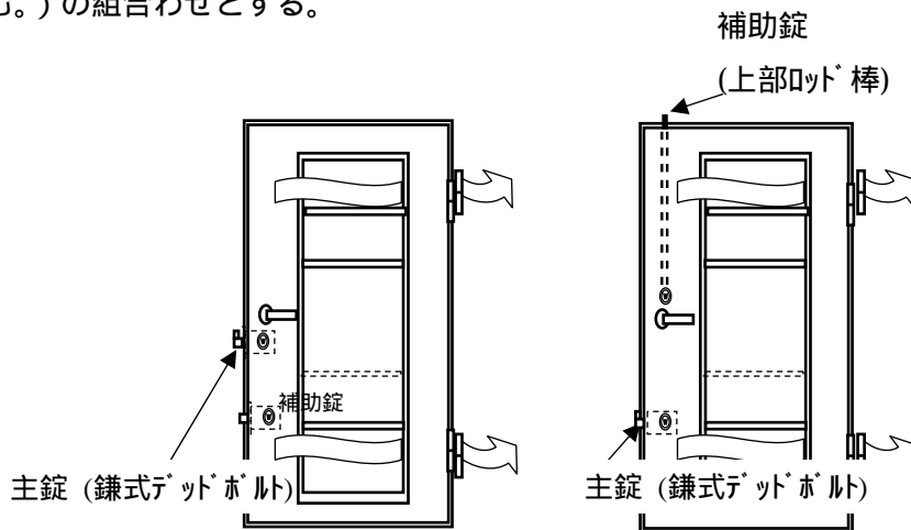
図4 - 1 上げ下げ内蔵ドア 扉本体の構造例
